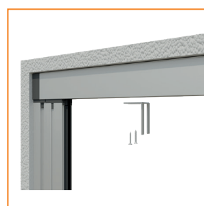
8. Fissare il fermo di battuta centrale all'interno della guida superiore
